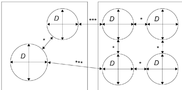
Tanks beliebig aufgestellt (4 Tanks in Gruppe)
