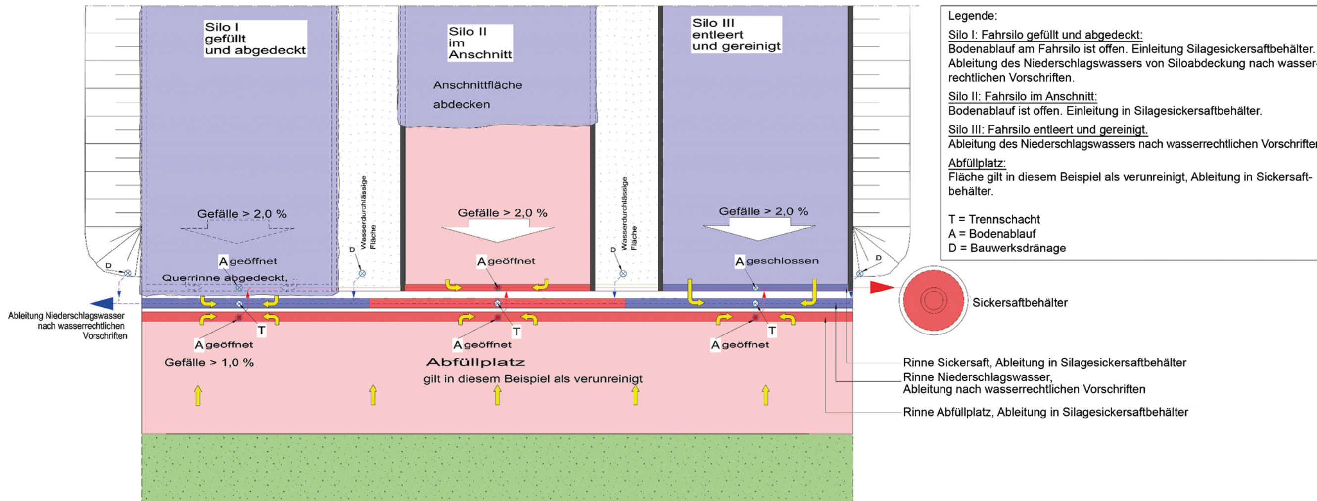
Gefälleschema Querrinne
