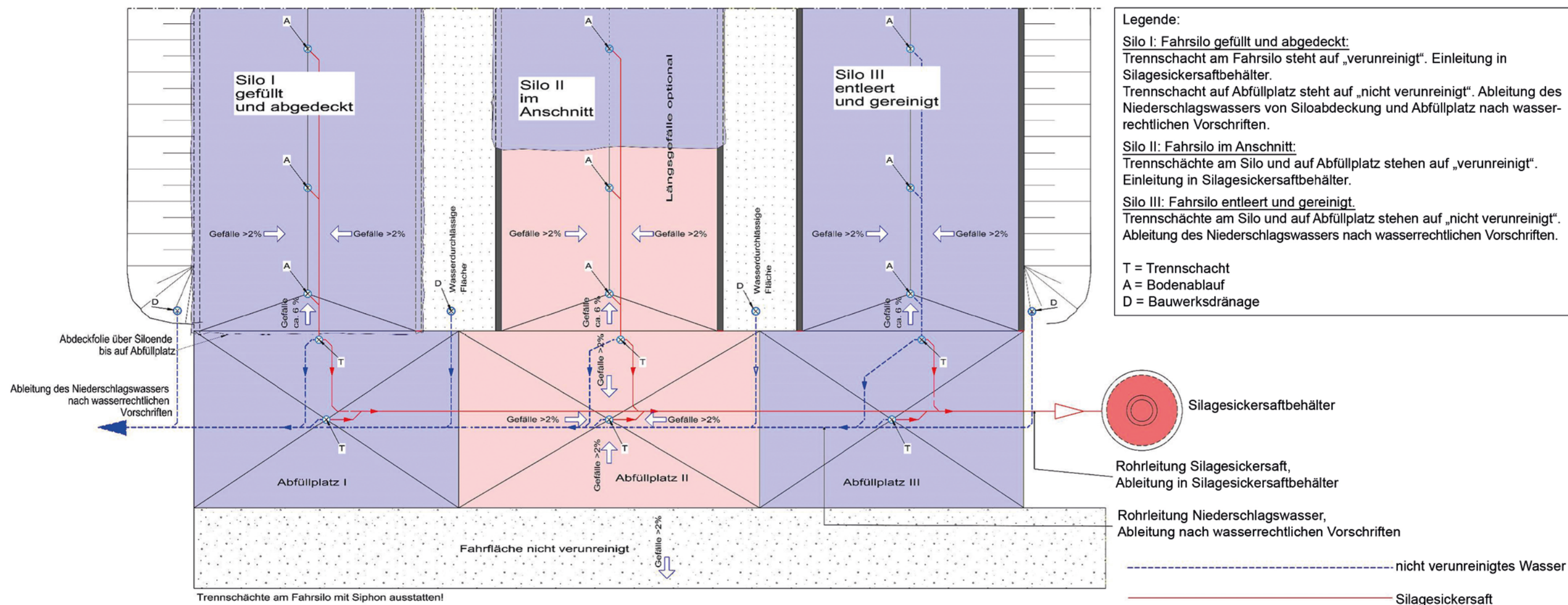
Grundriss
